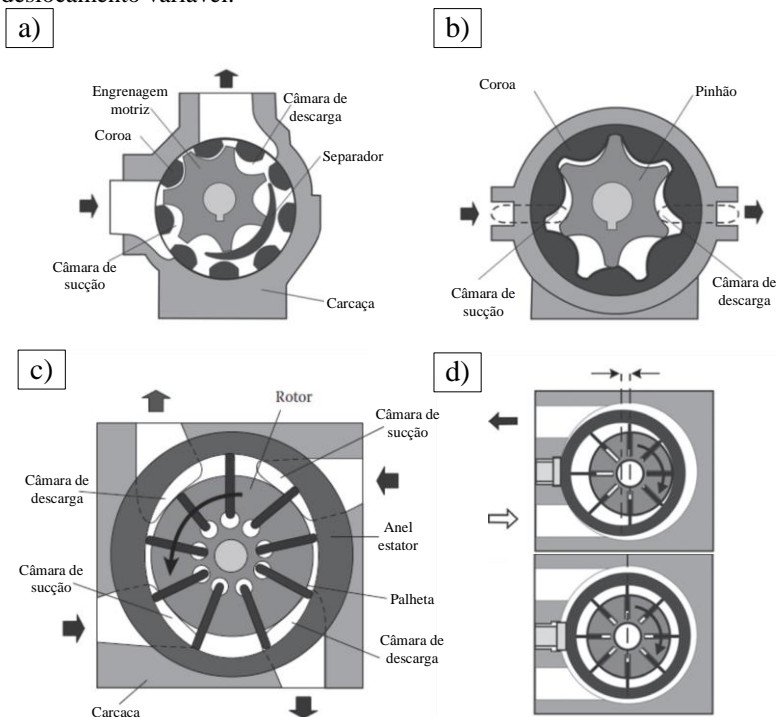
Figura 2.14 - Tipos comuns de bombas hidráulicas em transmissões automáticas: (a) engrenagens internas; (b) gerotor; (c) palhetas compensada; (d) palhetas com deslocamento variável.
