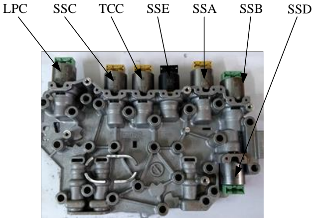
Figura 3.9 - Solenoides no corpo de válvulas.
