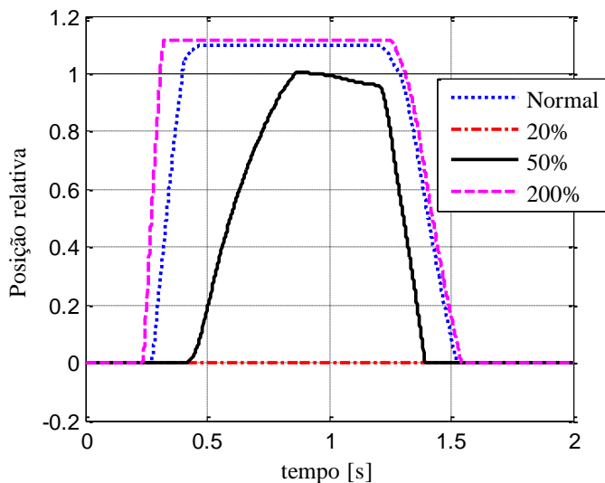
Figura 6.26 - Deslocamentos para análise de sensibilidade das pressões de suprimento.
